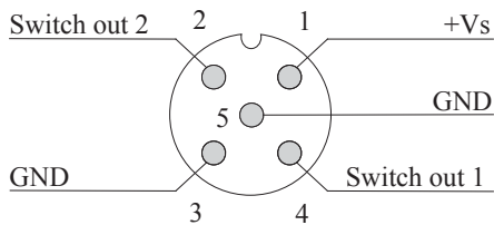
MIK-...E14R, MIK-...G14R Cable Connection
